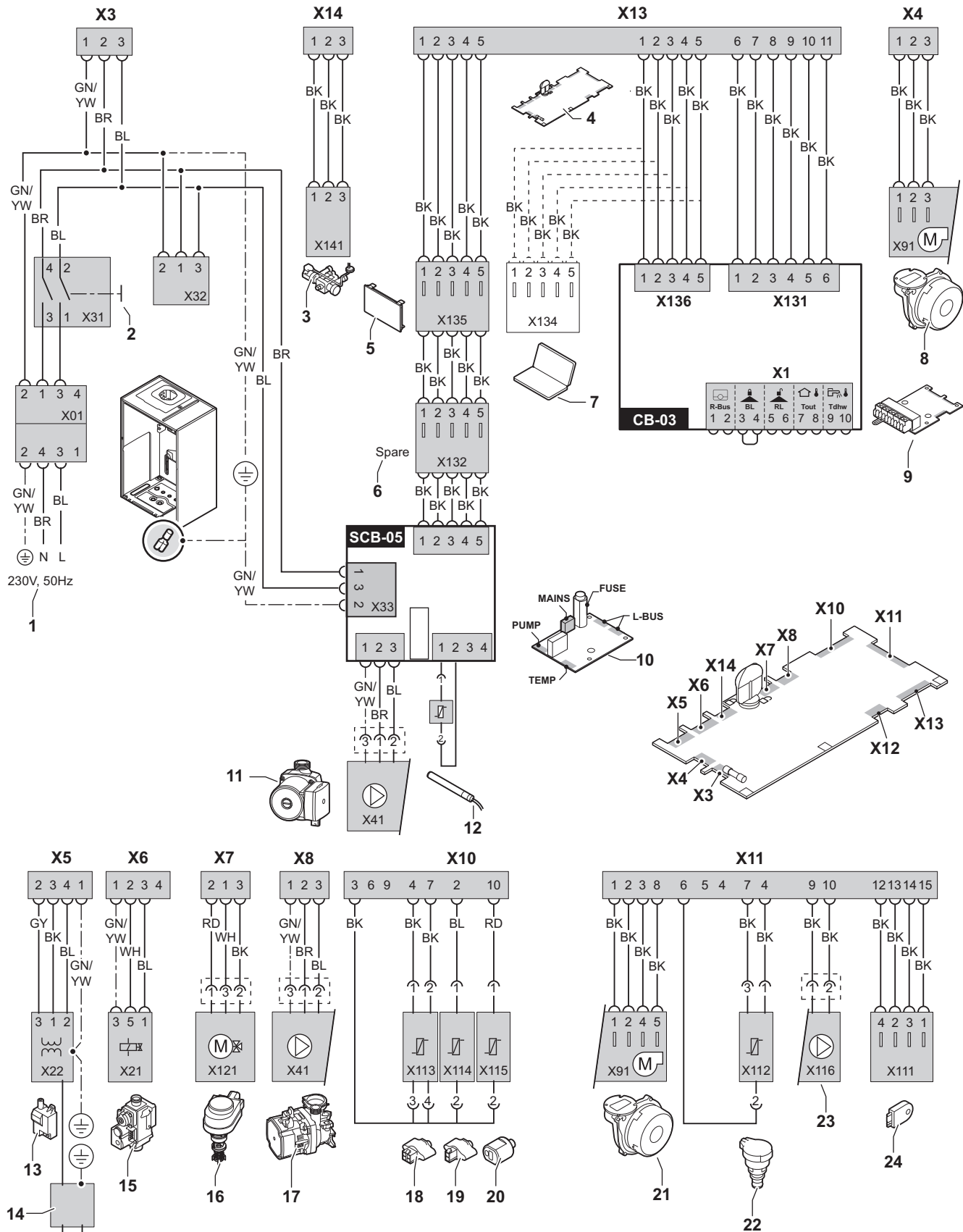
ábra2 Kapcsolási rajz
