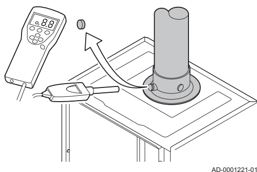
ábra21 Füstgázmérő csomak
