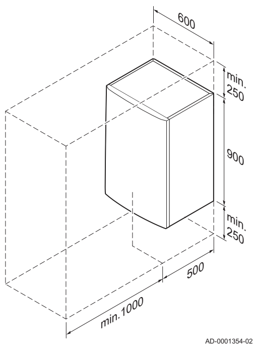
ábra7 Felszerelési terület
