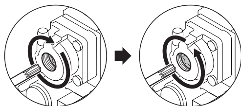
ábra34 B szabályozócsavar
