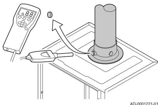
ábra26 Füstgázmérő csomak
