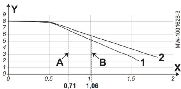
4. ábra Rendelkezésre álló nyomás
