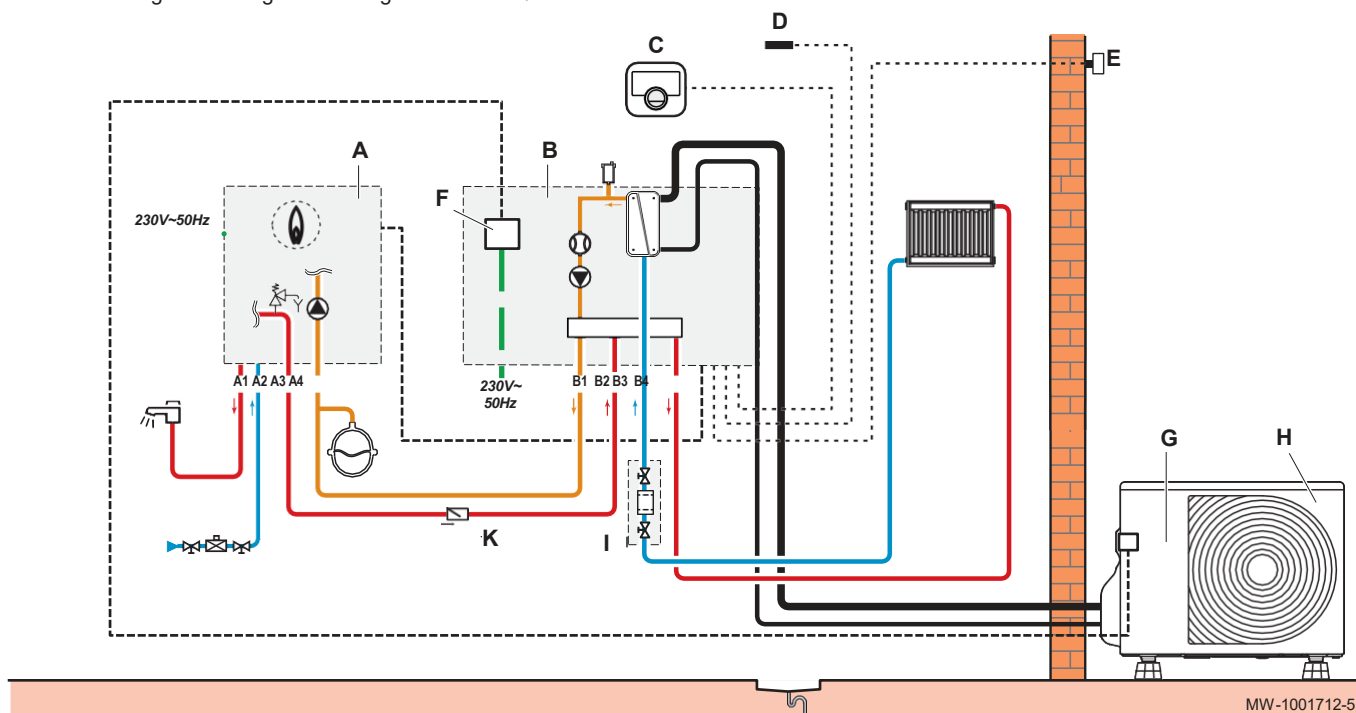
2. séma: túláram szeleppel és puffertartállyal ellátott rendszer
