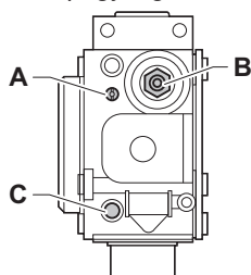
ábra42 Gázszelepegyeség
