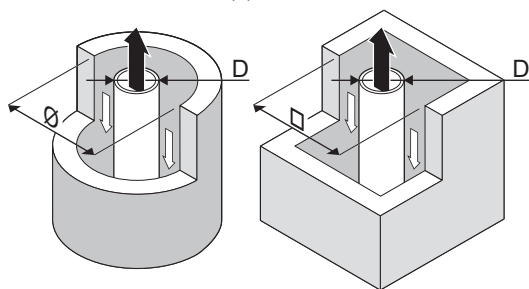
ábra3 Az akna vagy légszatórna mínimális mérete C_{93(X)}
