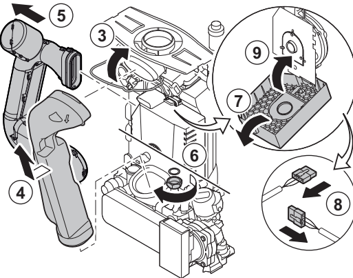
ábra67 Szétszerelés
