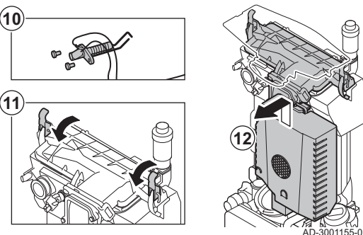
ábra67 Szétszerelés
