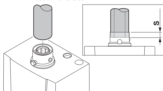
ábra18 Füstgázelvezető és levegőbemenet csatlakoztatása
