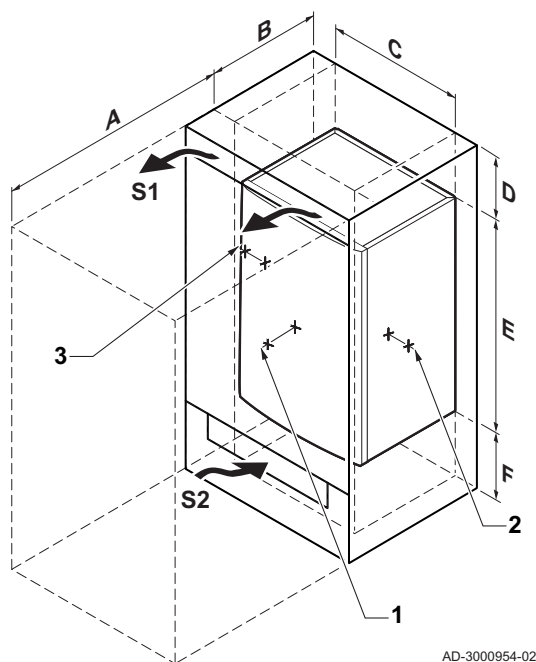
ábra3 Felszerelési terület
