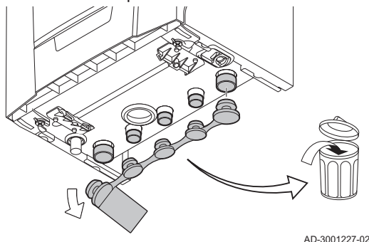
ábra17 Védősapkák levétele
