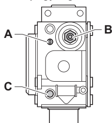
ábra45 Gázszelepegyeség
