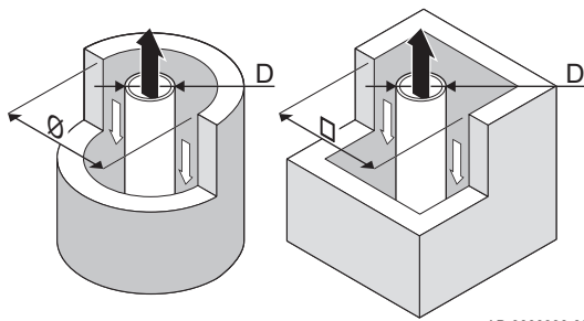
ábra4 Az akna vagy légcsonna minimális mérete C_{93(X)}
