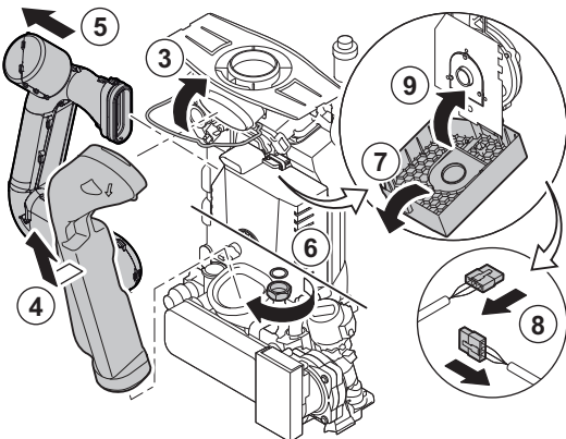
ábra68 Szétszerelés
