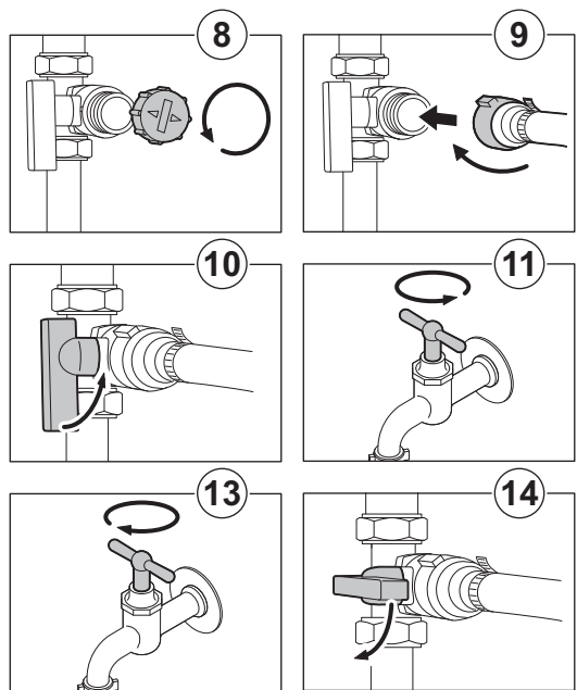
ábra85 A rendszer utántöltése
