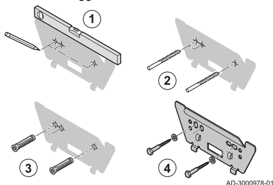
ábra16 A kazán felszerelése
