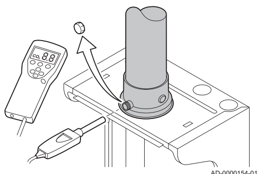
ábra40 Füstgázmérő csomak
